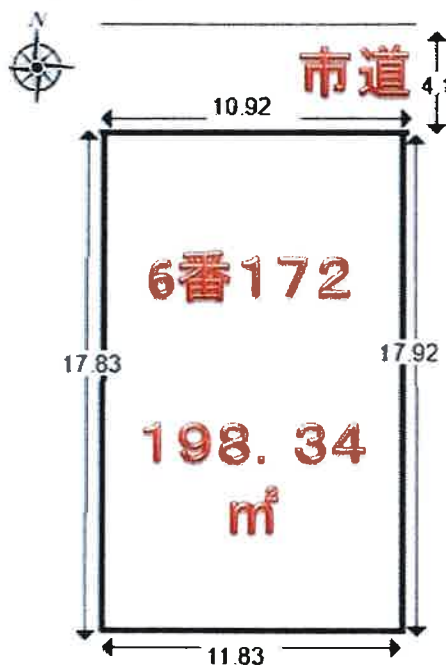
測量図
